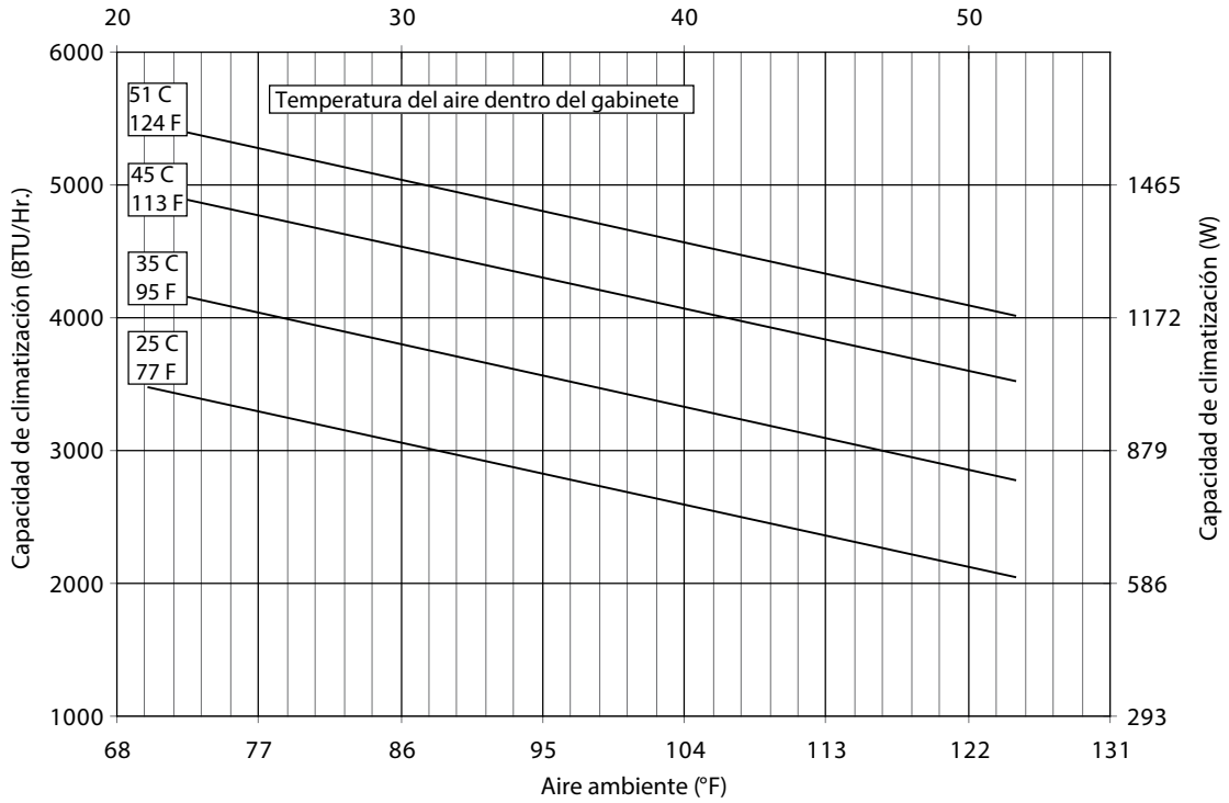
N28-0416-GXXX Curvas de capacidad a 60 Hz Aire ambiente (°C)
