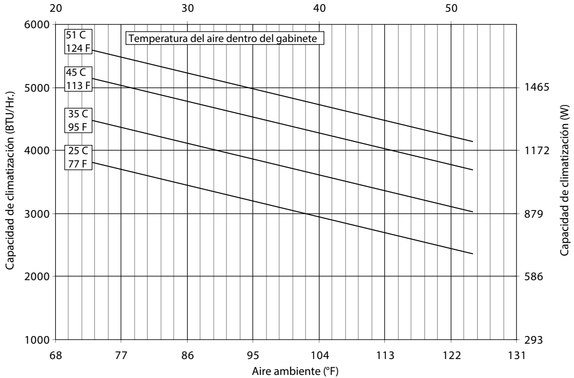
N28-0416-GXXX Curvas de capacidad a 60 Hz Aire ambiente (°C)
